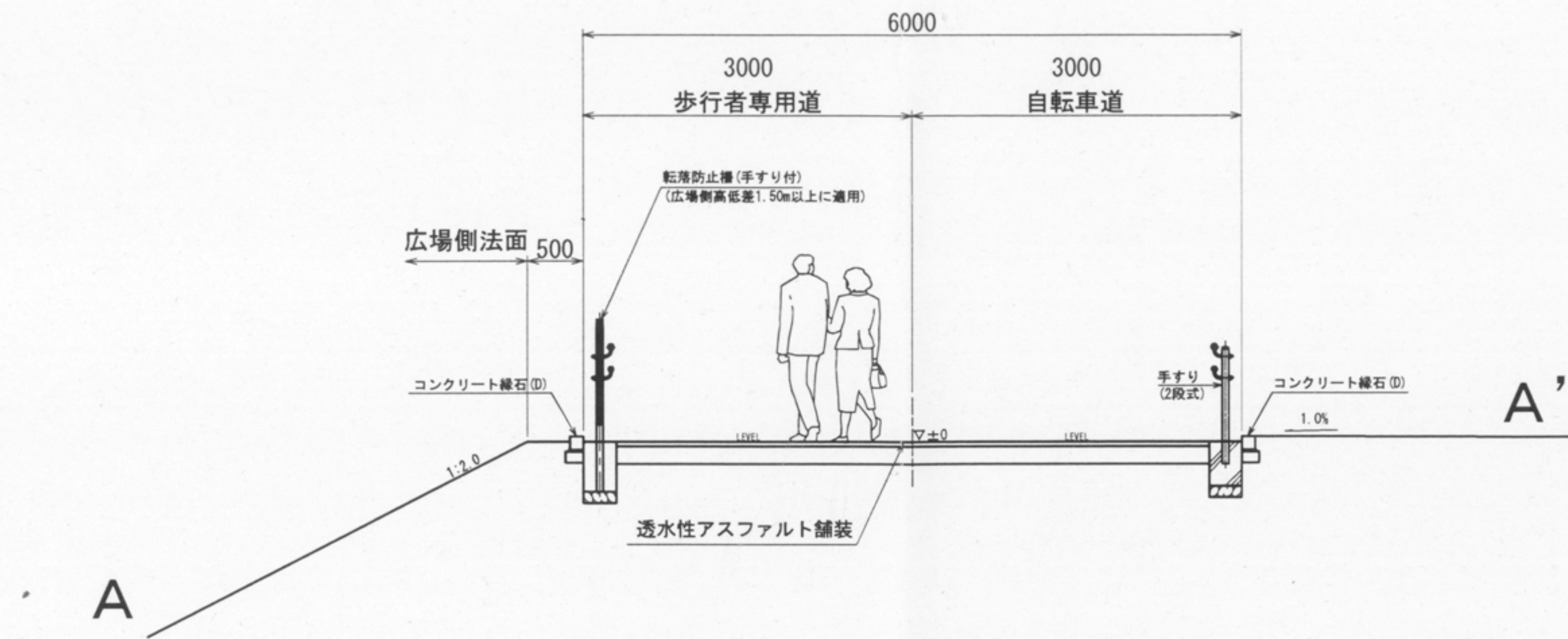
A-A' 断面図
