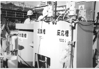
▲余水処理実験装置
